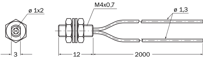
Rysunek wymiarowy
