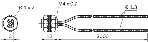
Rysunek wymiarowy LL3-DK66
