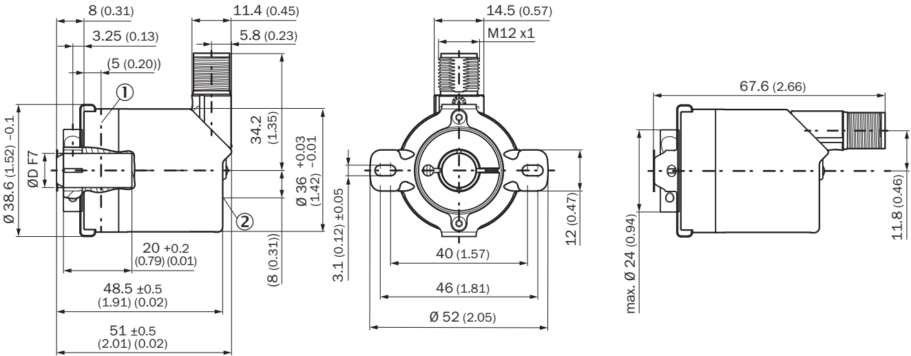
Wymiary w mm
