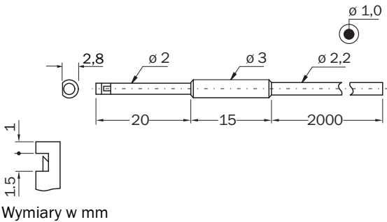
Rysunek wymiarowy
