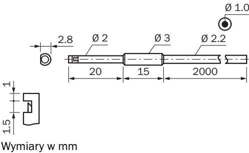
Rysunek wymiarowy LL3-TV01
