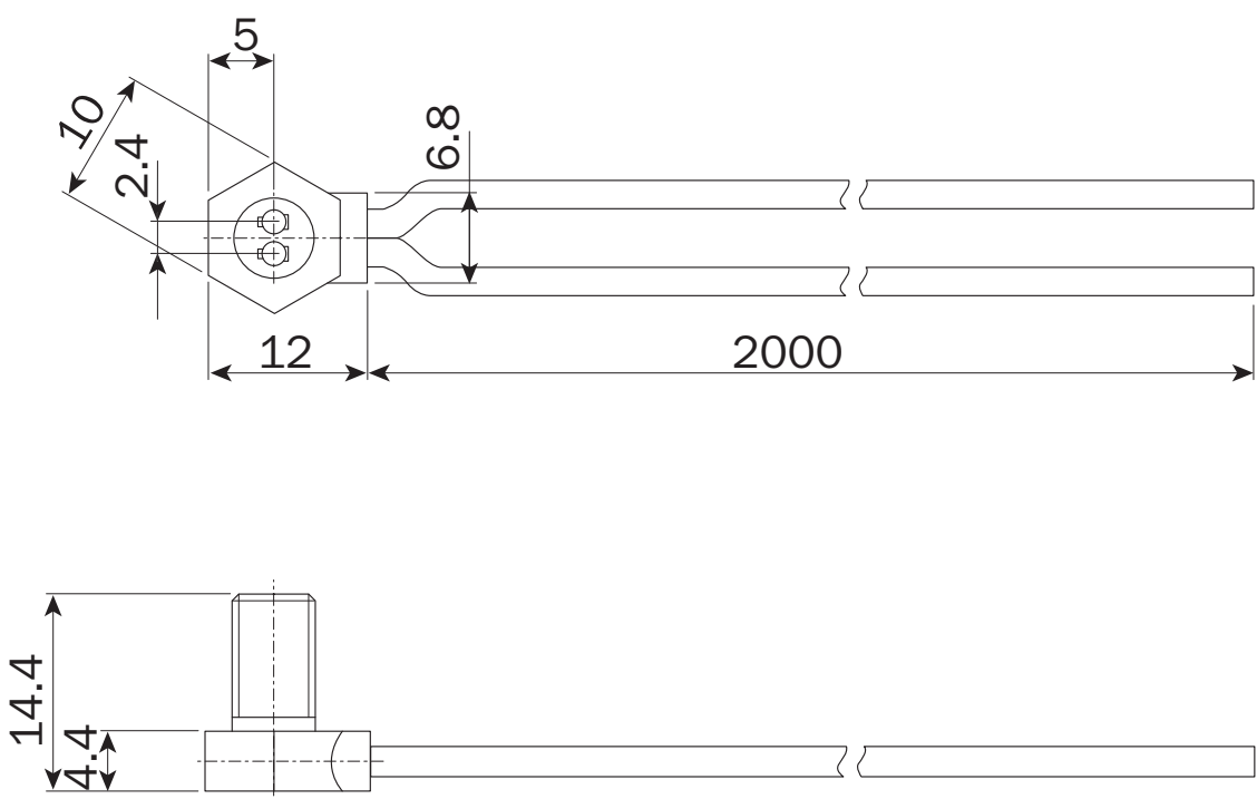
Rysunek wymiarowy LL3-DV05, LL3-DV06, LL3-DV07
