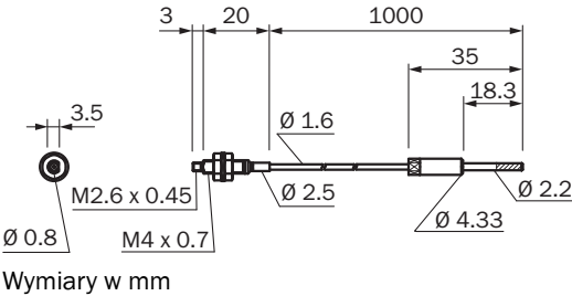
Rysunek wymiarowy LL3-TH10
