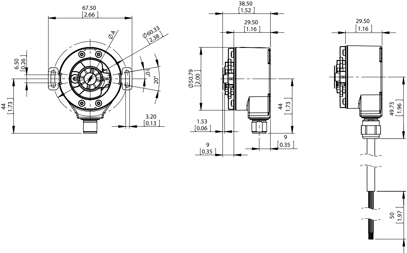
Rysunek wymiarowy DFS21 Otwór przelotowy
