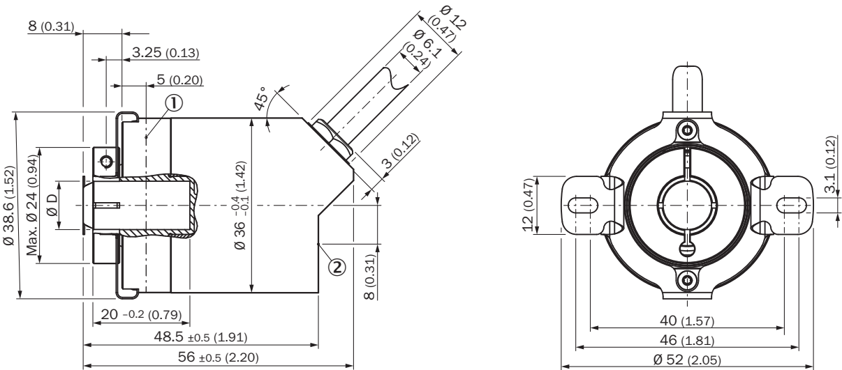
Rysunek wymiarowy Wersja z otworem nieprzelotowym, przewód
