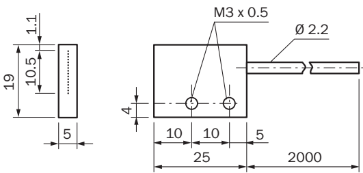
Rysunek wymiarowy LL3-TS14
