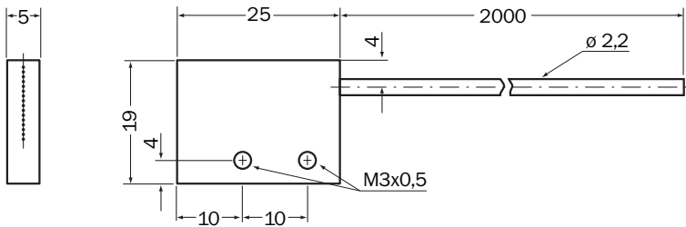
Rysunek wymiarowy
