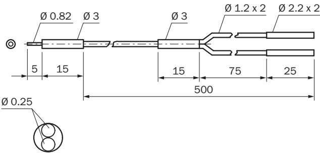
Rysunek wymiarowy LL3-DR05
