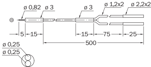
Rysunek wymiarowy
