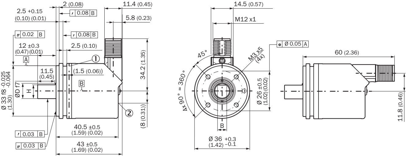
Wymiary w mm ① punkt pomiarowy temperatury roboczej ② punkt pomiarowy drgań
