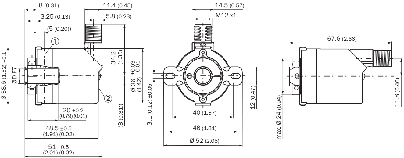
Rysunek wymiarowy Otwór nieprzelotowy, wtyk
