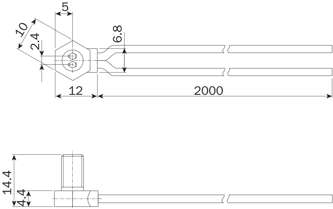
Rysunek wymiarowy LL3-DV05, LL3-DV06, LL3-DV07
