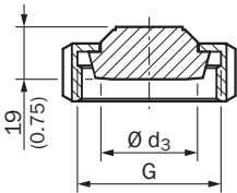
Rysunek wymiarowy Króciec stożkowy (DIN 11851) z rowkową nakrętką kołpakową
