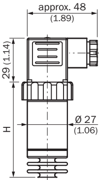
Rysunek wymiarowy Obudowa z wtykiem kątowym (DIN 175301-803 A), IP65
