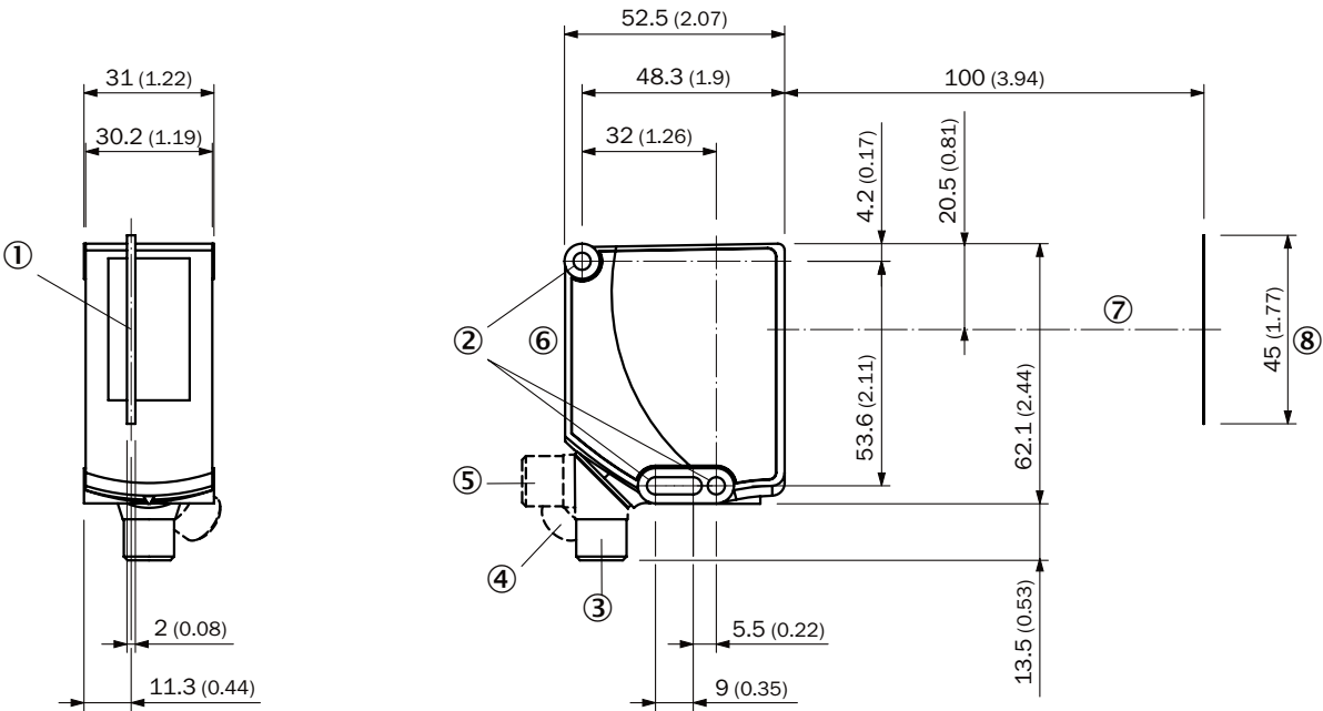
Rysunek wymiarowy AS30-xxx43xxxxxxxx
