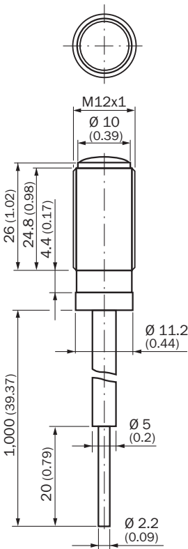
Rysunek wymiarowy LL3-TX02-01
