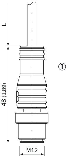
rysunek wymiarowy, przyłącze
