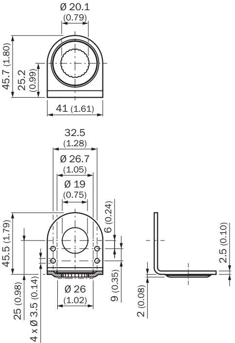
Wymiary w mm
