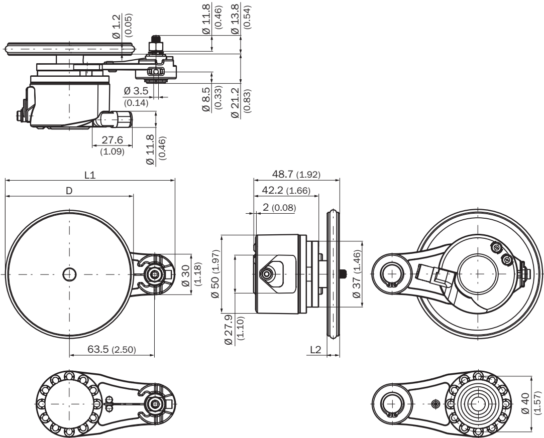
Rysunek wymiarowy Koło pomiarowe, ramię sprężynowe 63,5 mm, koło pomiarowe po stronie montażu, wtyk
