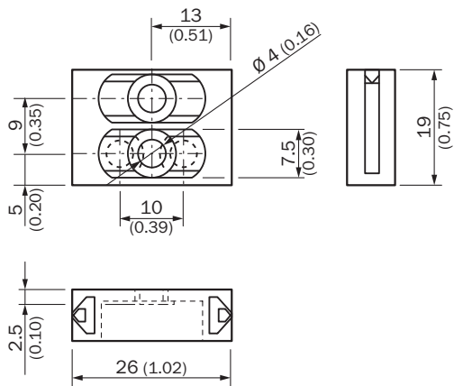
rysunek wymiarowy: BEF-SLG2
