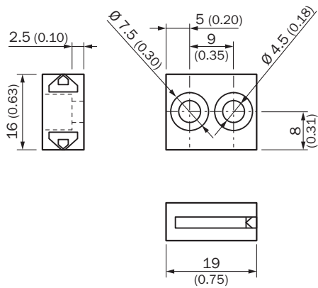
rysunek wymiarowy: BEF-SLG1
