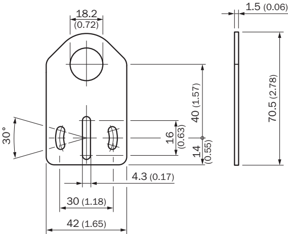
Rysunek wymiarowy
