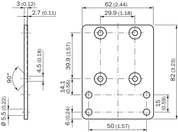
Rysunek wymiarowy
