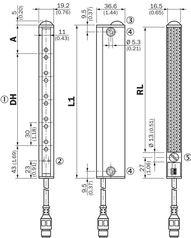
Rysunek wymiarowy PLG3
