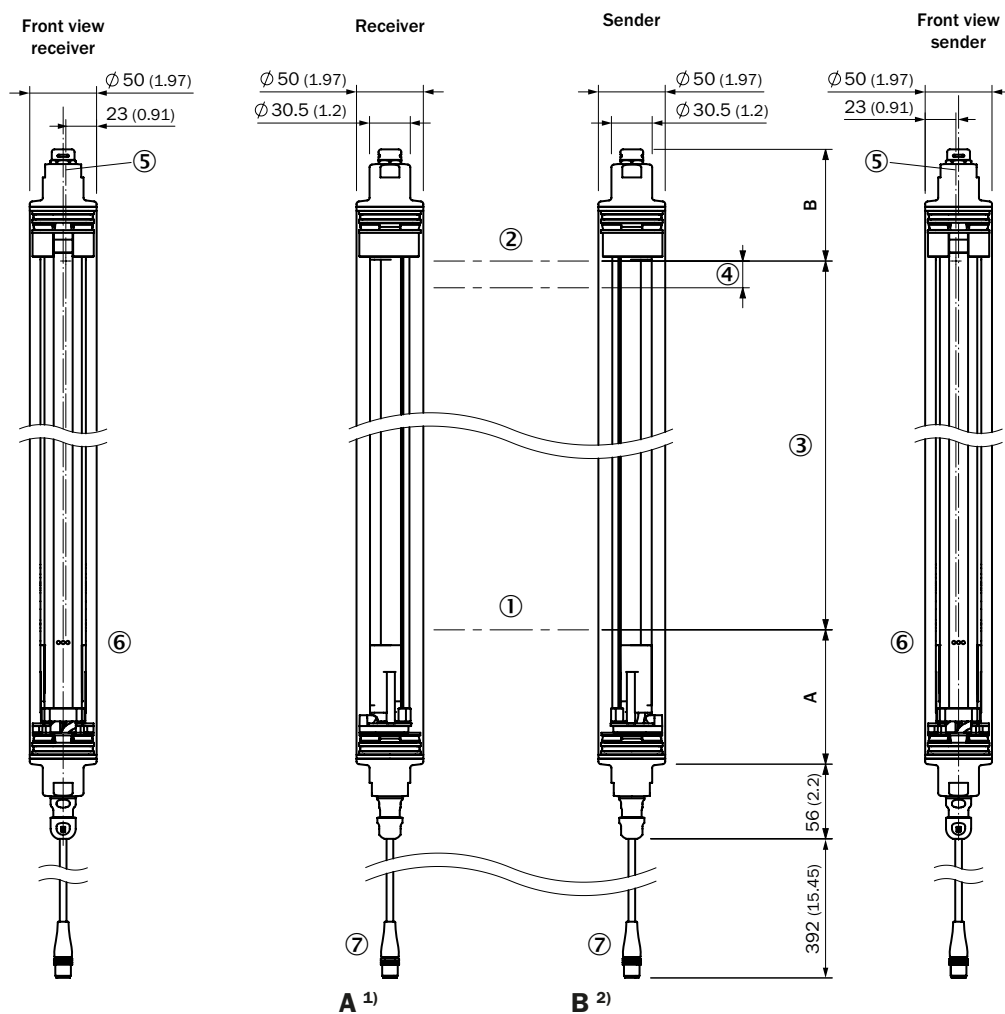
Rysunek wymiarowy
