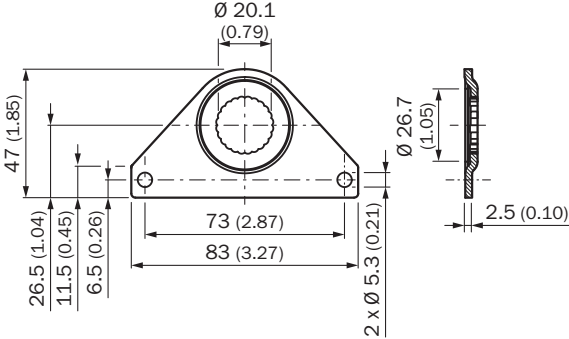
Rysunek wymiarowy
