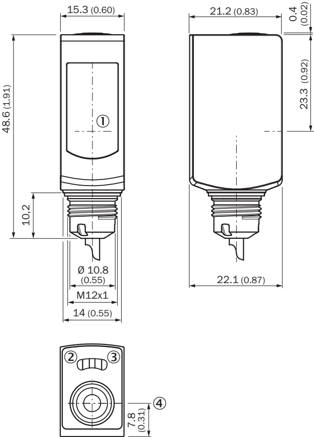
Wymiary w mm
