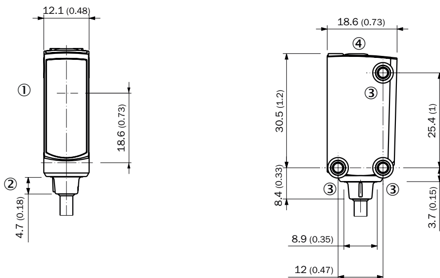
Rysunek wymiarowy, czujnik
