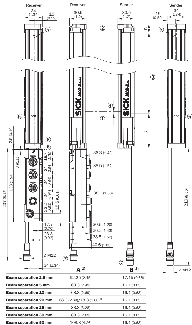
Rysunek wymiarowy
