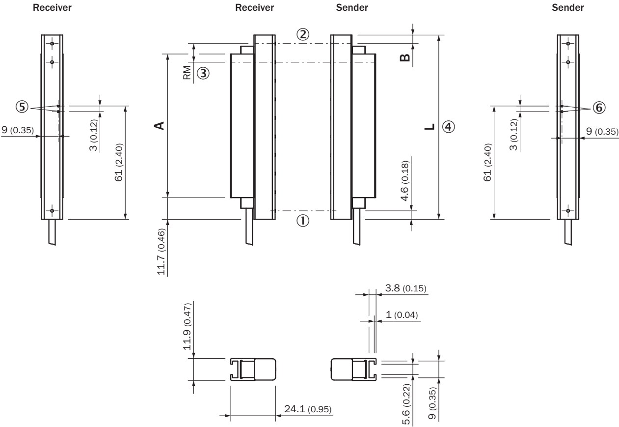
Rysunek wymiarowy, czujnik
