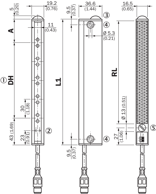
Rysunek wymiarowy PLG3
