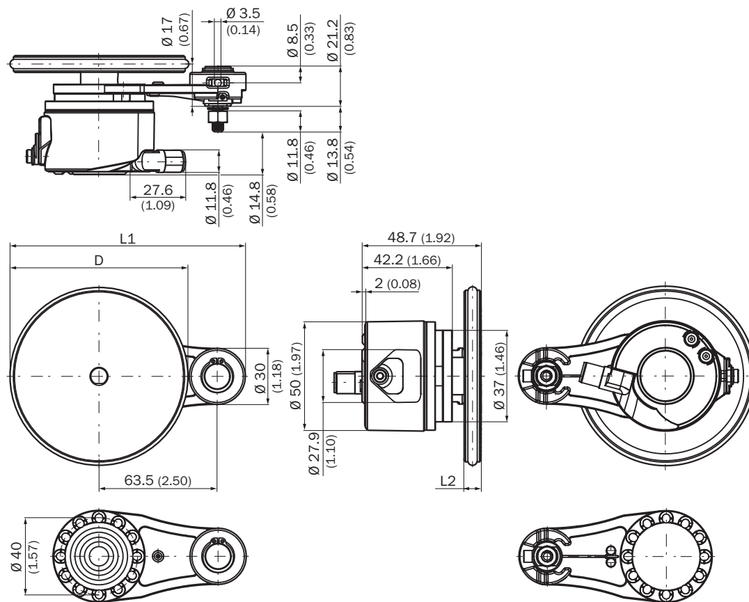
Rysunek wymiarowy Koło pomiarowe, ramię sprężynowe 63,5 mm, enkoder po stronie montażu, wtyk
