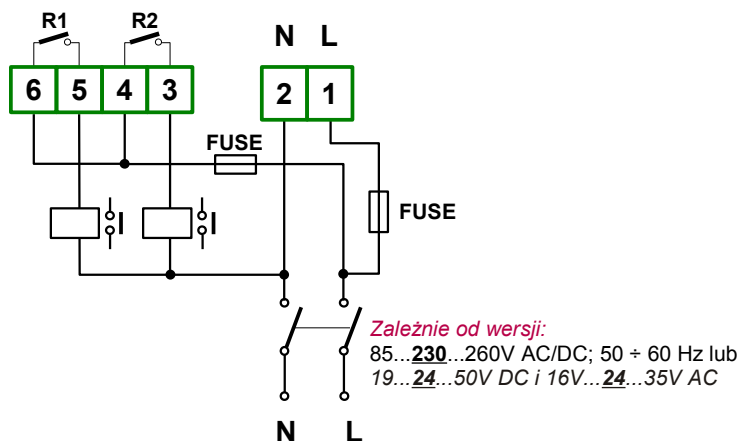
Rys. 4.6. Podłączenie zasilania oraz przekaźników sterujących obciążeniami
