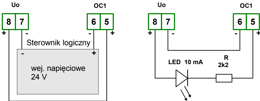
Rys. 4.8. Przykładowe podłączenia wyjścia typu OC
