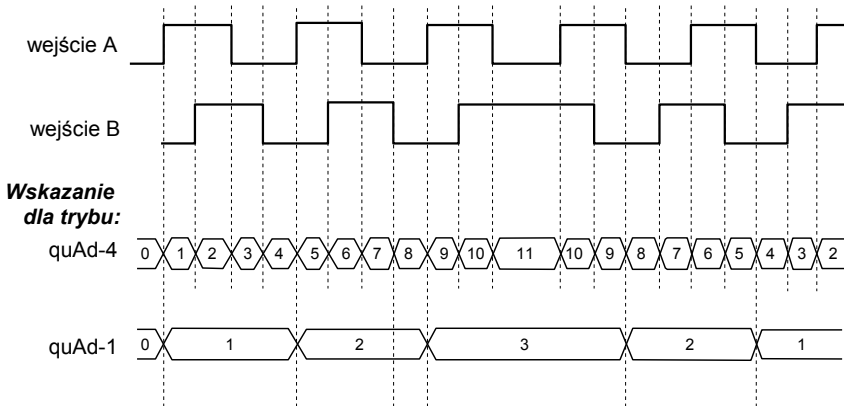
Rys. 6.1. Sposób naliczania w licznikach serii SLIK (przy ustawach muL ="1", div ="1", OFFSEt ="0"): a) w trybach " A+B ", " A-B "; b) w trybach " quAd-4 ", " quAd-1 "
