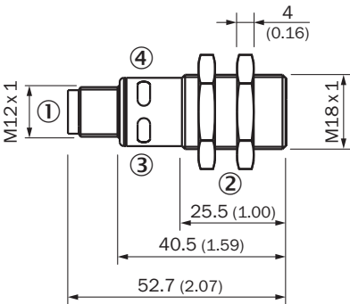
Rysunek wymiarowy UM18-2xxxxx1
