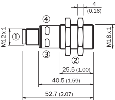
Rysunek wymiarowy UM18-2xxxxx1
