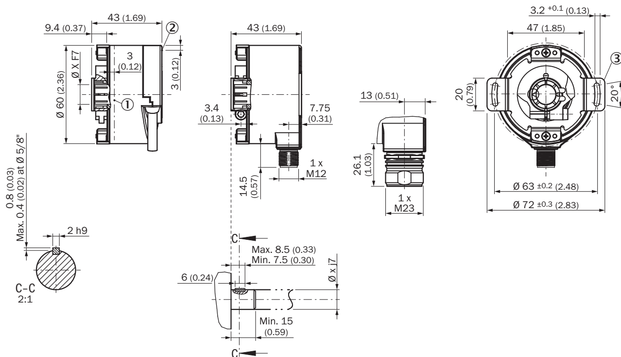
Rysunek wymiarowy Wersja z otworem nieprzelotowym – system zorientowany na bezpieczeństwo
