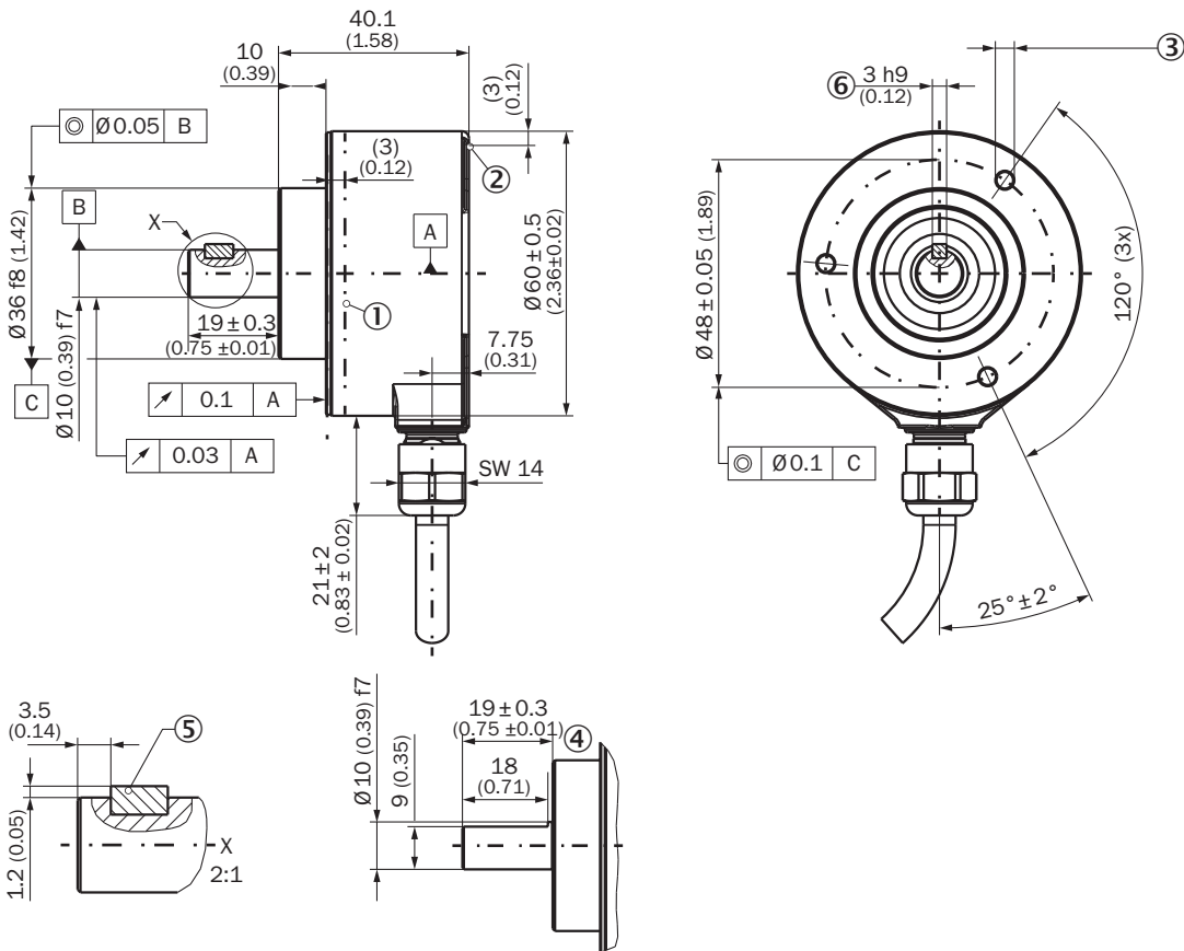
Rysunek wymiarowy Wałek, mocowanie czołowe, przewód promieniowy
