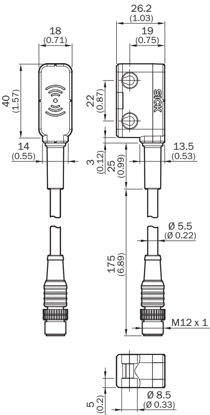
Rysunek wymiarowy Czujnik z przewodem i wtykiem
