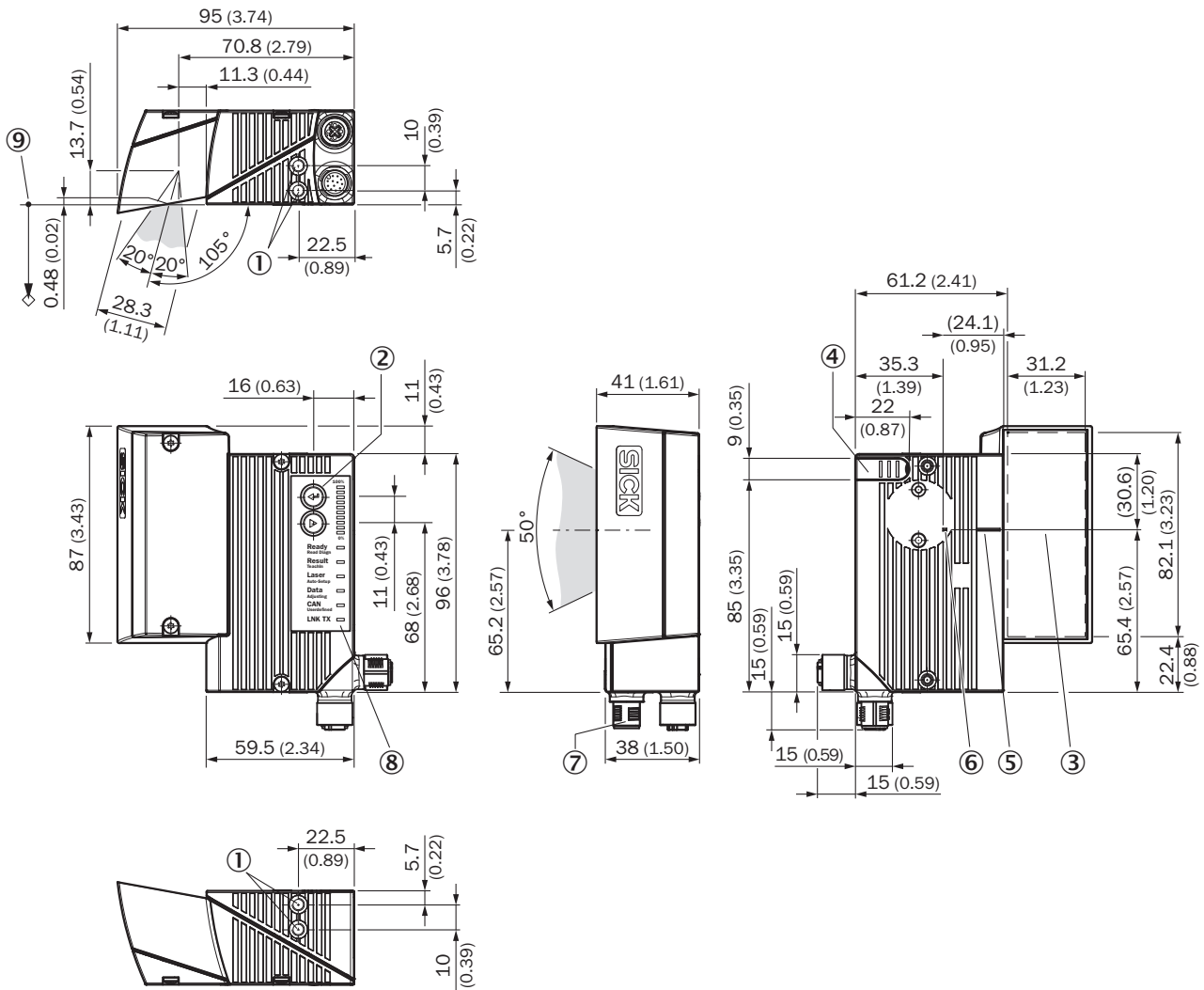
Rysunek wymiarowy CLV63x/64x/65x, JEF3xx, JEF5xx, Ethernet, wahiwe lustro
