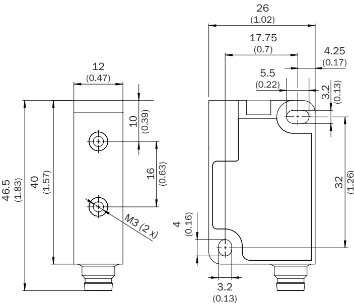
Wymiary w mm
