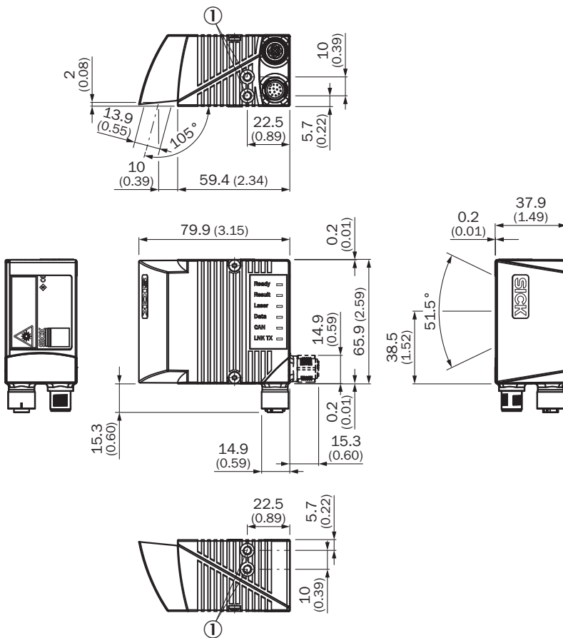
Rysunek wymiarowy CLV62x Ethernet, z boku
