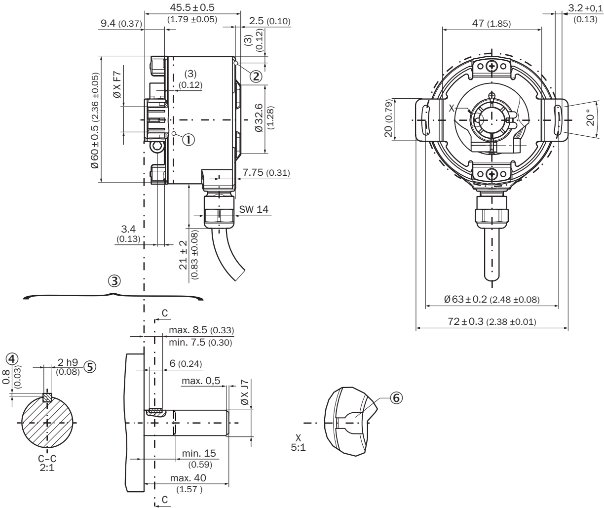
Rysunek wymiarowy Otwór nieprzelotowy, przewód promieniowy
