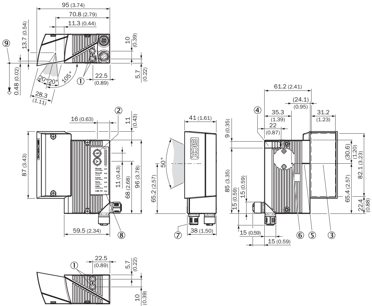
Rysunek wymiarowy CLV63x/64x/65x, JEF3xx, JEF5xx, Ethernet, wahlwe lustro
