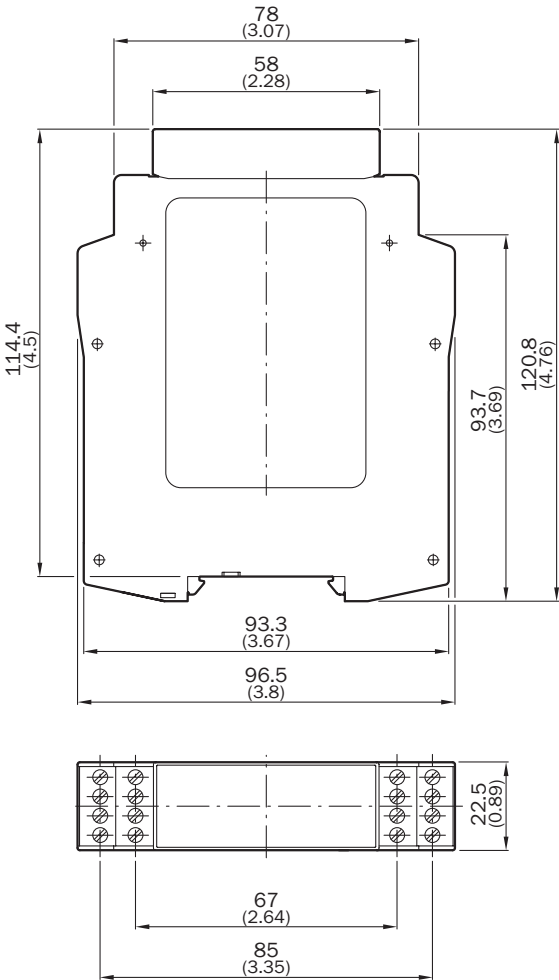
Rysunek wymiarowy Moduł główny Flexi Classic
