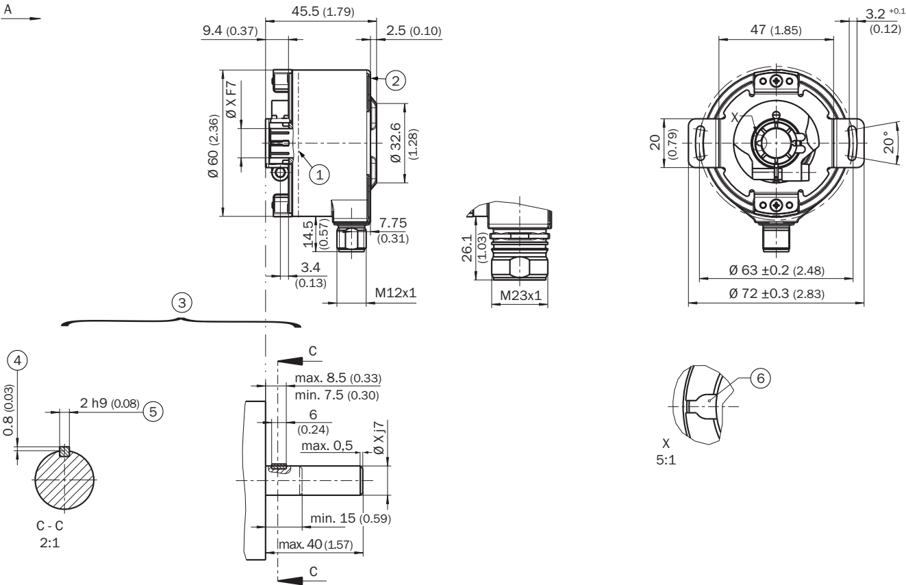
Rysunek wymiarowy Otwór nieprzelotowy, wtyk promieniowy M12 i M23
