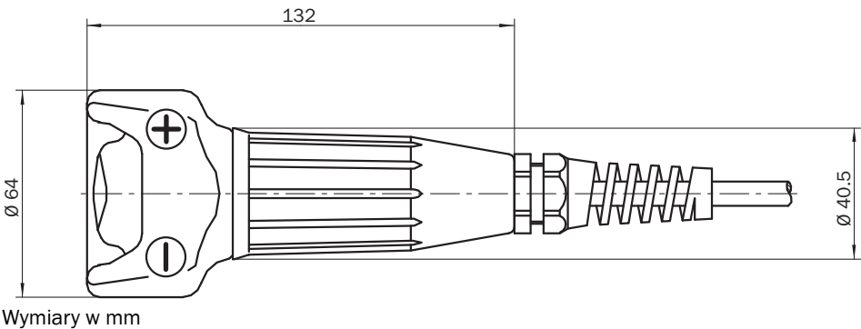
Rysunek wymiarowy E100-B
