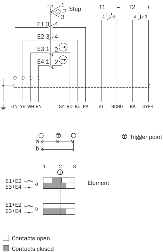
Wykres drogi przełączania E100-B
