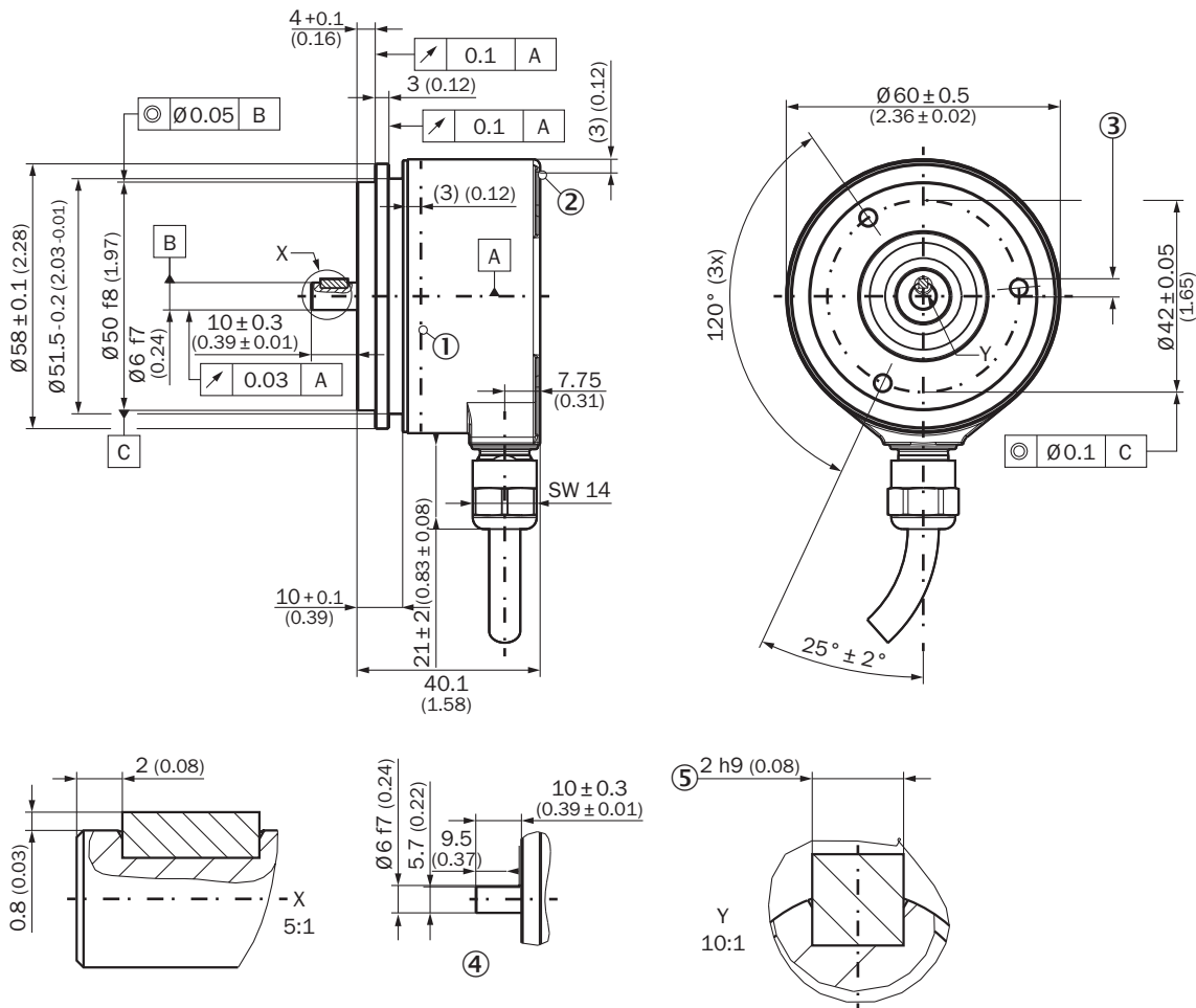
Rysunek wymiarowy Wałek, mocowanie na serwokółnierzu, przewód promieniowy
