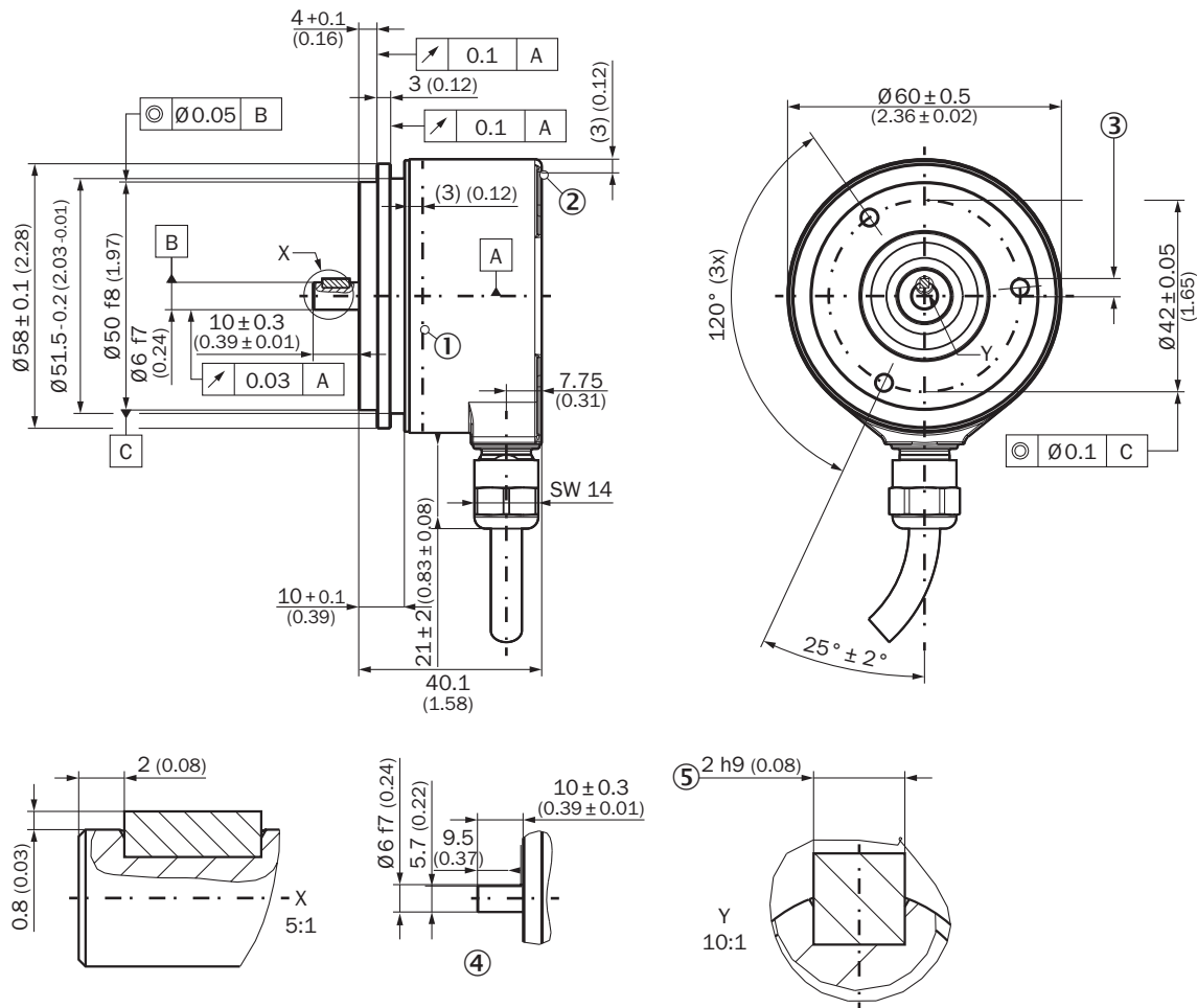
Rysunek wymiarowy Wałek, mocowanie na serwokołnierzu, przewód promieniowy
