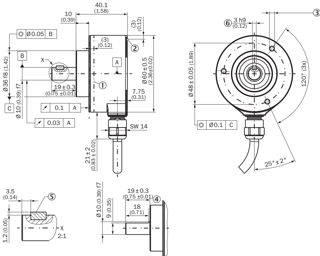
Rysunek wymiarowy Wałek, mocowanie czołowe, przewód promieniowy
