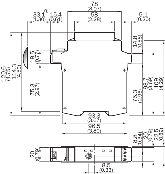
Rysunek wymiarowy FX3-CPU1, FX3-CPU2
