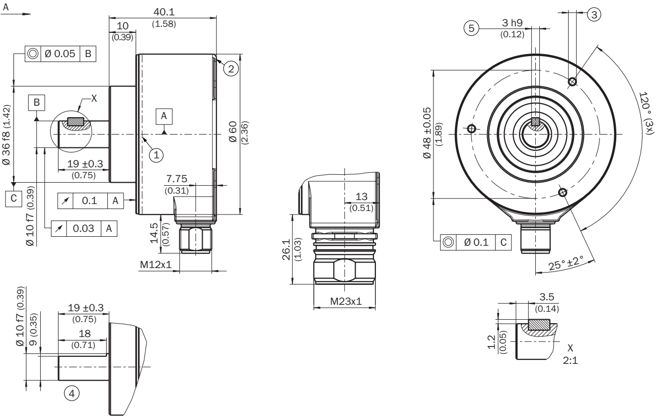
Rysunek wymiarowy Wałek, mocowanie czołowe, wtyk promieniowy M12 i M23
