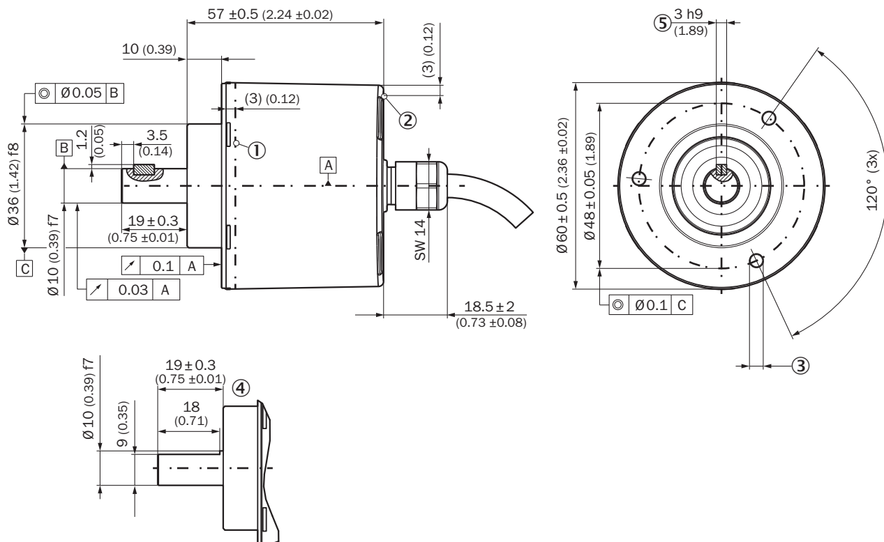
Rysunek wymiarowy Walek, mocowanie czołowe, przewód osiowy
